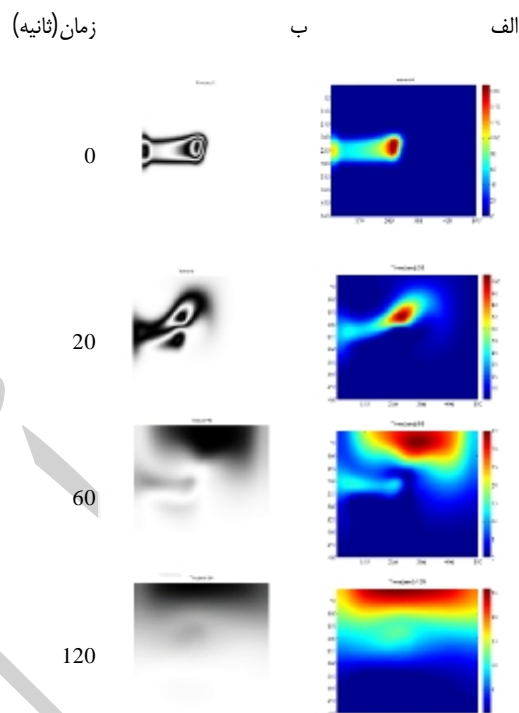
شکل 7. نیم رخ دز جذب شده برای تابش پروتونی 40 MeV از وجه جانبی. الف) توزیع دمایی معادل توزیع دز در ماده جاذب و ب) نوارهای تداخلی ناشی از جذب دز در ماده که توسط دوربین کالریمتر ثبت و بازسازی شده است که نماینده نواحی هم دز در ماده تحت تابش یونساز است.
