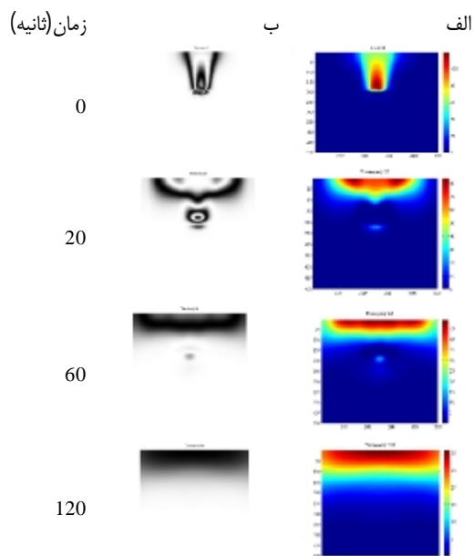
شکل 8. نیم رخ دز جذب شده برای تابش پروتونی 40 MeV از وجه بالا. الف) توزیع دمایی معادل توزیع دز در ماده جاذب و ب) نوارهای تداخلی ناشی از جذب دز در ماده که توسط دوربین کالریمتر ثبت و بازسازی شده است که نماینده نواحی هم دز در ماده تحت تابش یونساز است.
