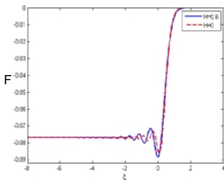
شکل 5. جواب معادله (7) به ازای مقادیر مختلف H
