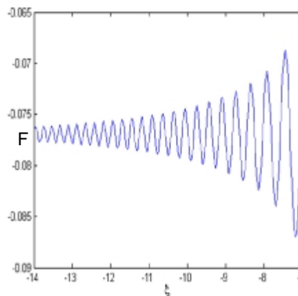
شکل 4. جواب معادله (7) به ازای مقادیر مختلف H
