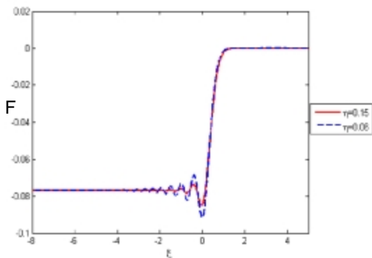
شکل 2. جواب نوسانی موج ضربه
