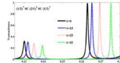
نمودار 5. طیف تراگسیل فیلتر دو کاناله برای مقادیر مختلف زاویه موج تابشی پرتو گاوسی با مختصه شعاعی r = 2\text{mm}
